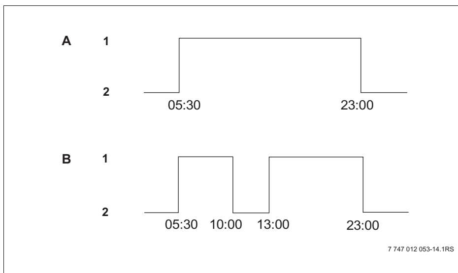
Obr. 16 Vložení spínacích bodů k přerušení fáze vytápění
