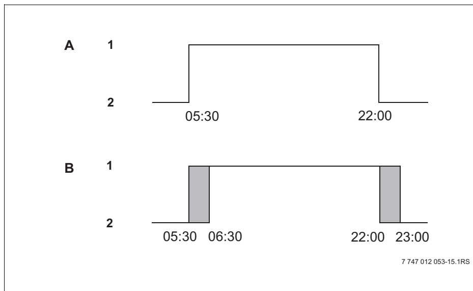
Obr. 14 Změna spínacího bodu z 05:30 na 06:30 hod a z 22:00 na 23:00 hod (příklad)
