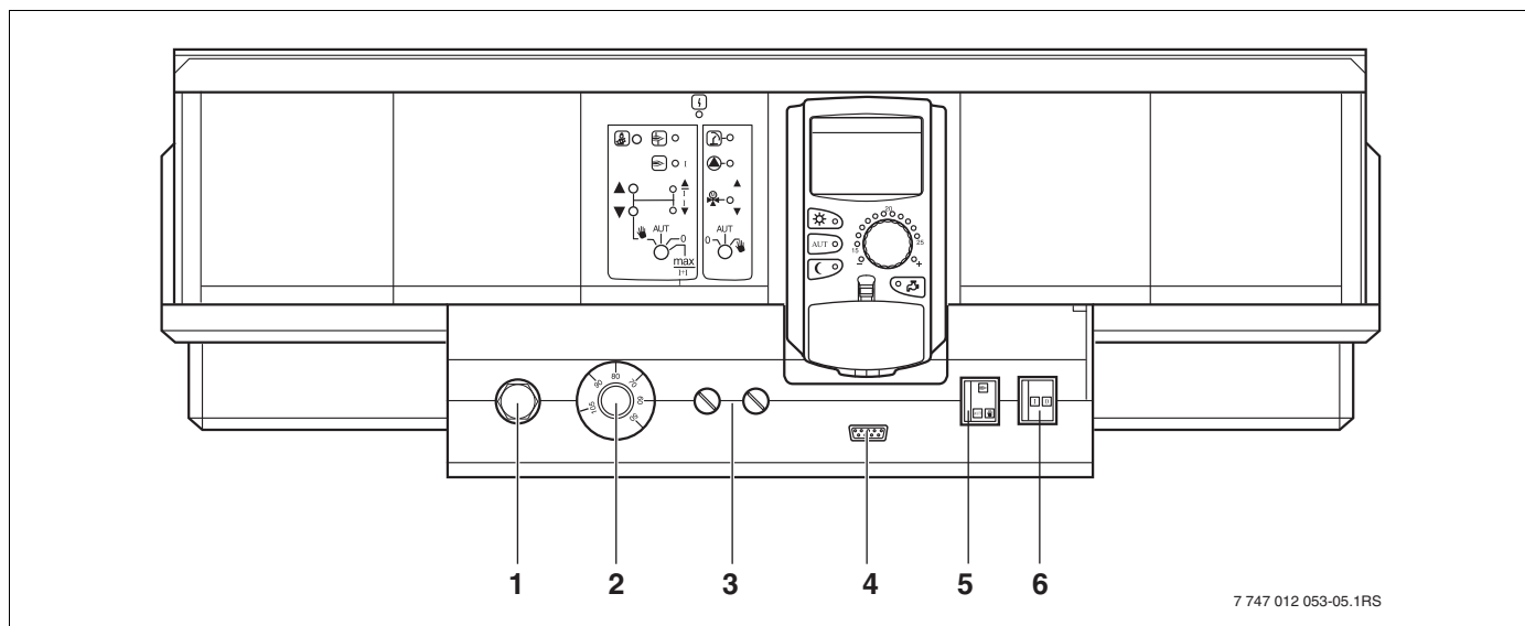
Obr. 4 Ovládací prvky regulačního přístroje Logamatic 4321 - (stav při expedici)
