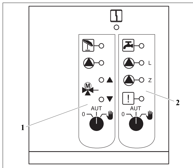
Obr. 22 Funkční modul FM441
