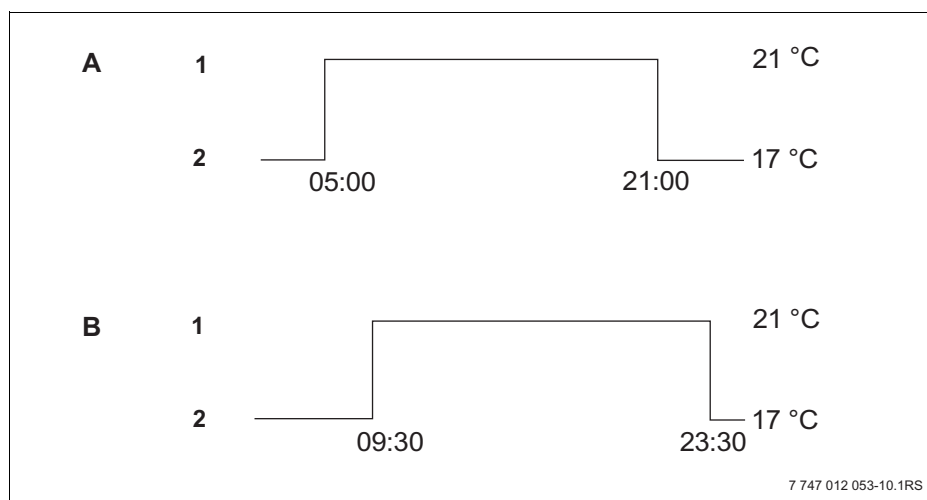
Obr. 20 Nový vytápěcí program
