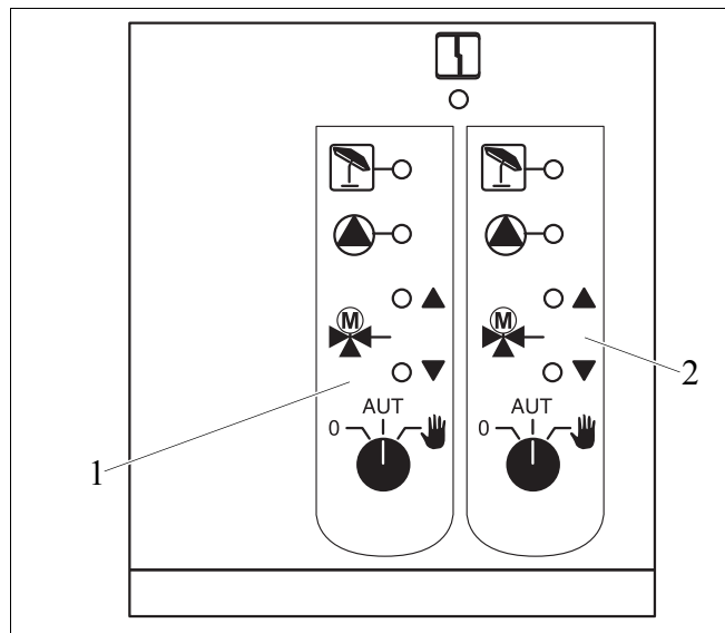
Obr. 24 Funkční modul FM442
