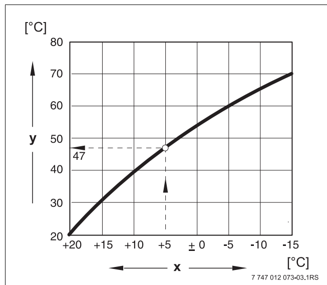
Obr. 3 Topná křivka vytápěcího okruhu (příklad)
